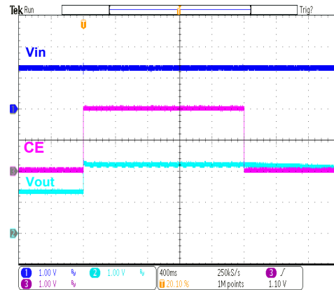
HT7722B Chip Enable/Disable
