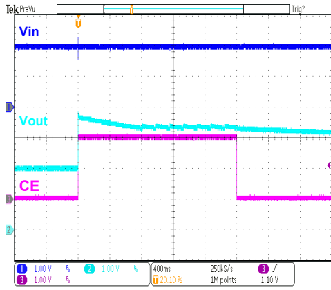
HT7733B Chip Enable/Disable
