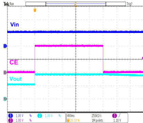
HT7718B Chip Enable/Disable
