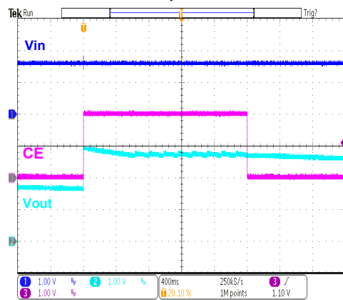
HT7727B Chip Enable/Disable
