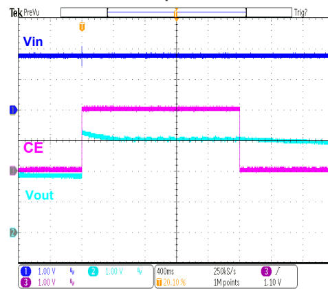
HT7730B Chip Enable/Disable
