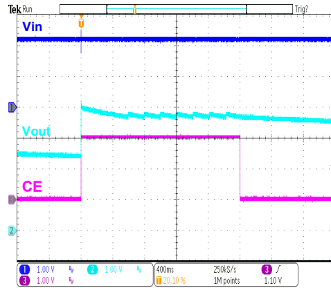
HT7737B Chip Enable/Disable
