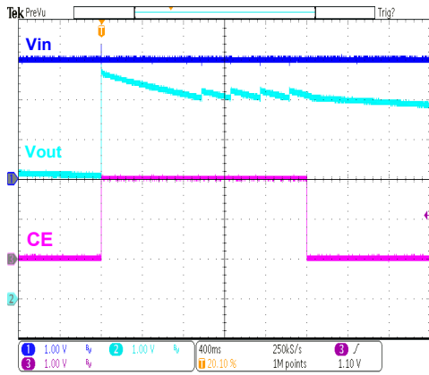
HT7750B Chip Enable/Disable
