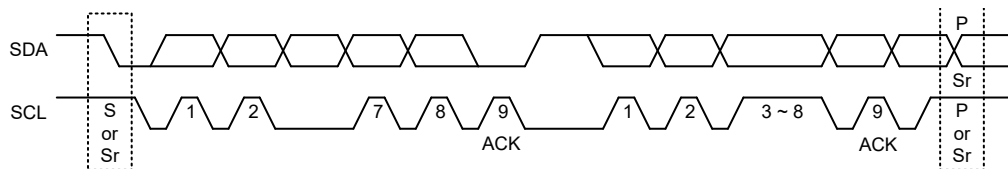
Figure 7. Byte Format
