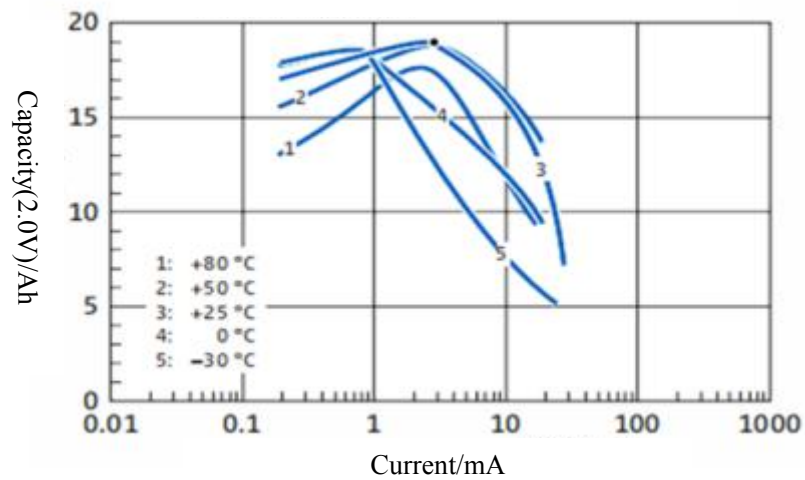
Capacity-Current Curve 容量-电流曲线
