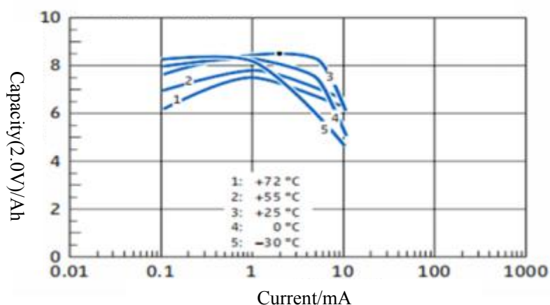
Capacity-Current Curve 容量-电流曲线
